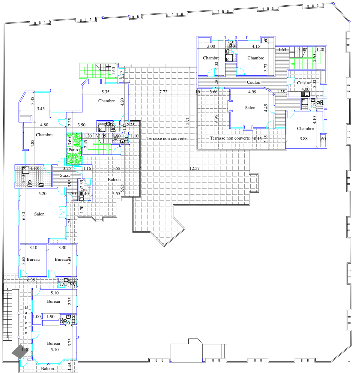
PLAN ETAGE EXISTANT
