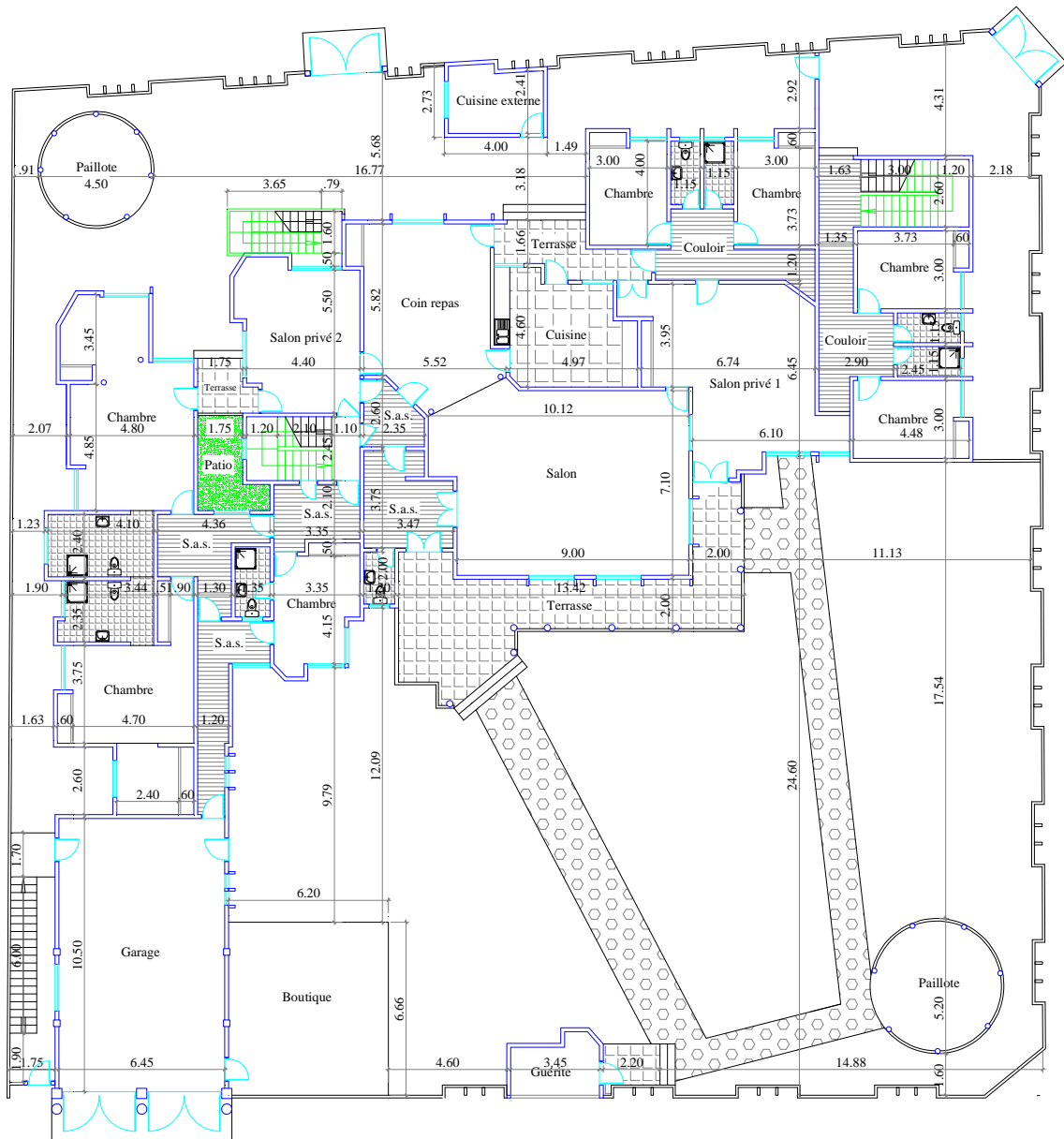
PLAN RDC ETATS DES LIEUX
